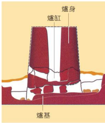
▲圖 2-9 鼓風豎爐剖面圖。戰國時期發明的鼓風豎爐，以高溫淬鍊出雜質少的液態鐵水，冷卻後再鑄成優質鐵器，這種冶鐵技術歐洲要到 14~15 世紀才發明。
